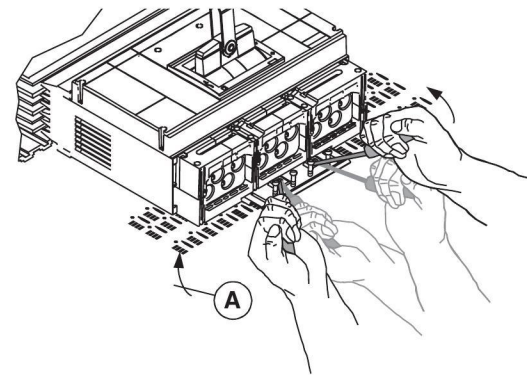
Figura 6: Inserción del interruptor automático en la barra
